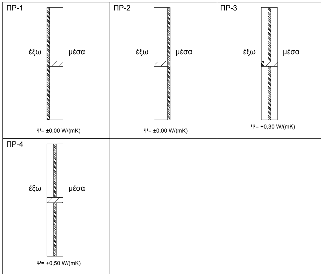
Πίνακας 16i. Θερμογέφυρες περιδέσμου ενίσχυσης.
