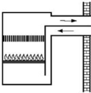
C 12 με ανεμιστήρα μετά τον εναλλάκτη θερμότητας
